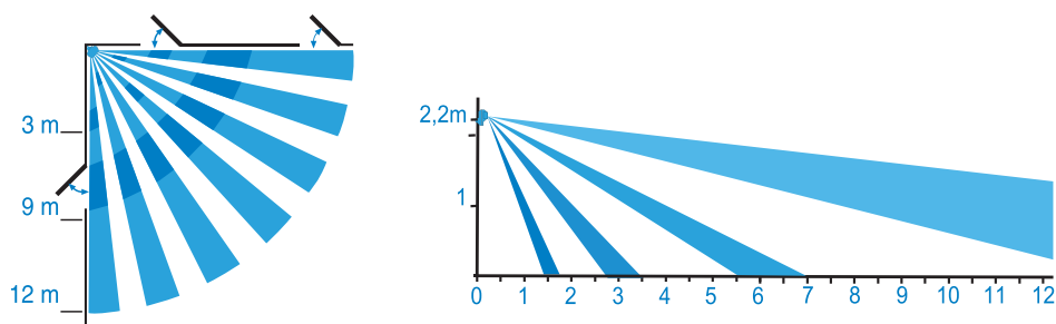
Schématisation des faisceaux de détection
